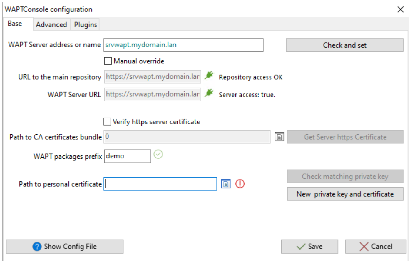
FIG. 13 – L'onglet basique pour les options de configuration de la console WAPT
