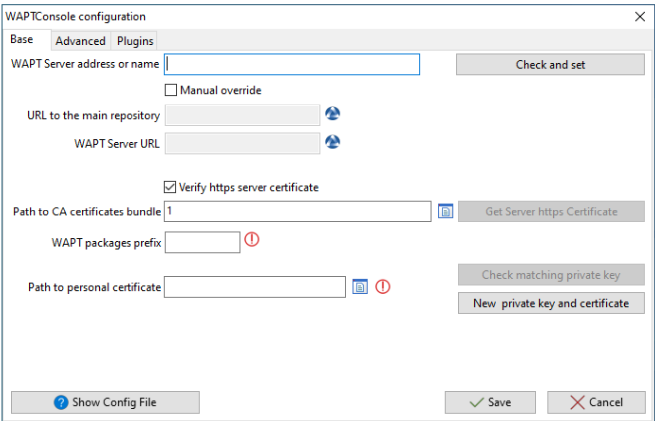
FIG. 10 – La fenêtre d'authentification de la console WAPT
