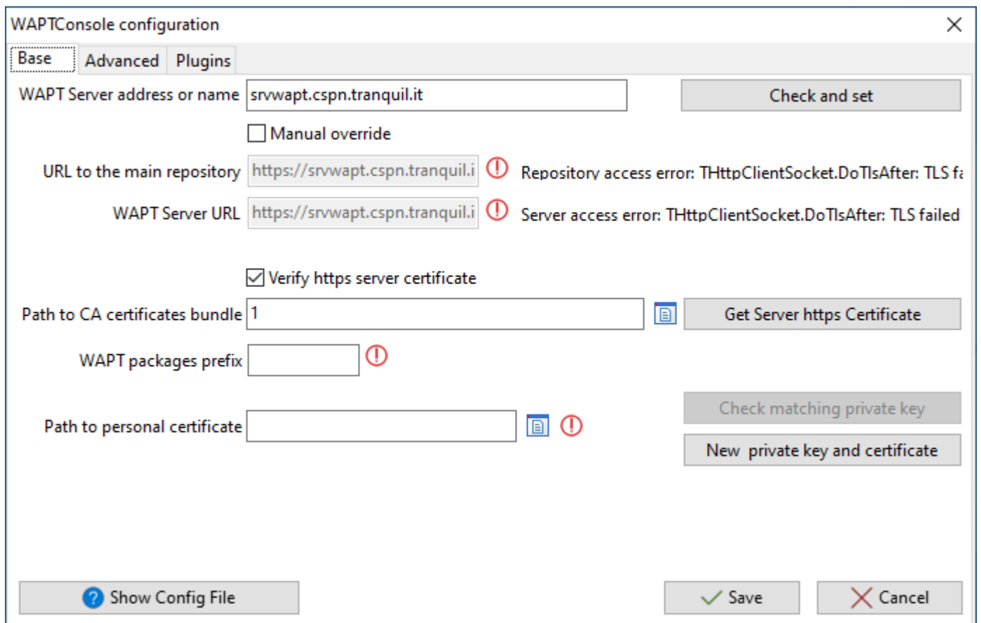
FIG. 6 – Erreur TLS dans la configuration de la console WAPT.
