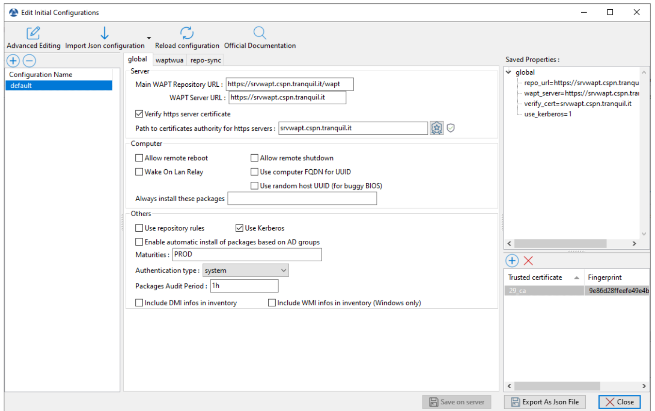
FIG. 29 – Éditer la configuration initiale
