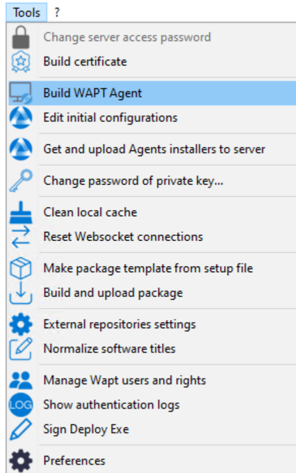
FIG. 21 – Générer l'agent WAPT depuis la console
