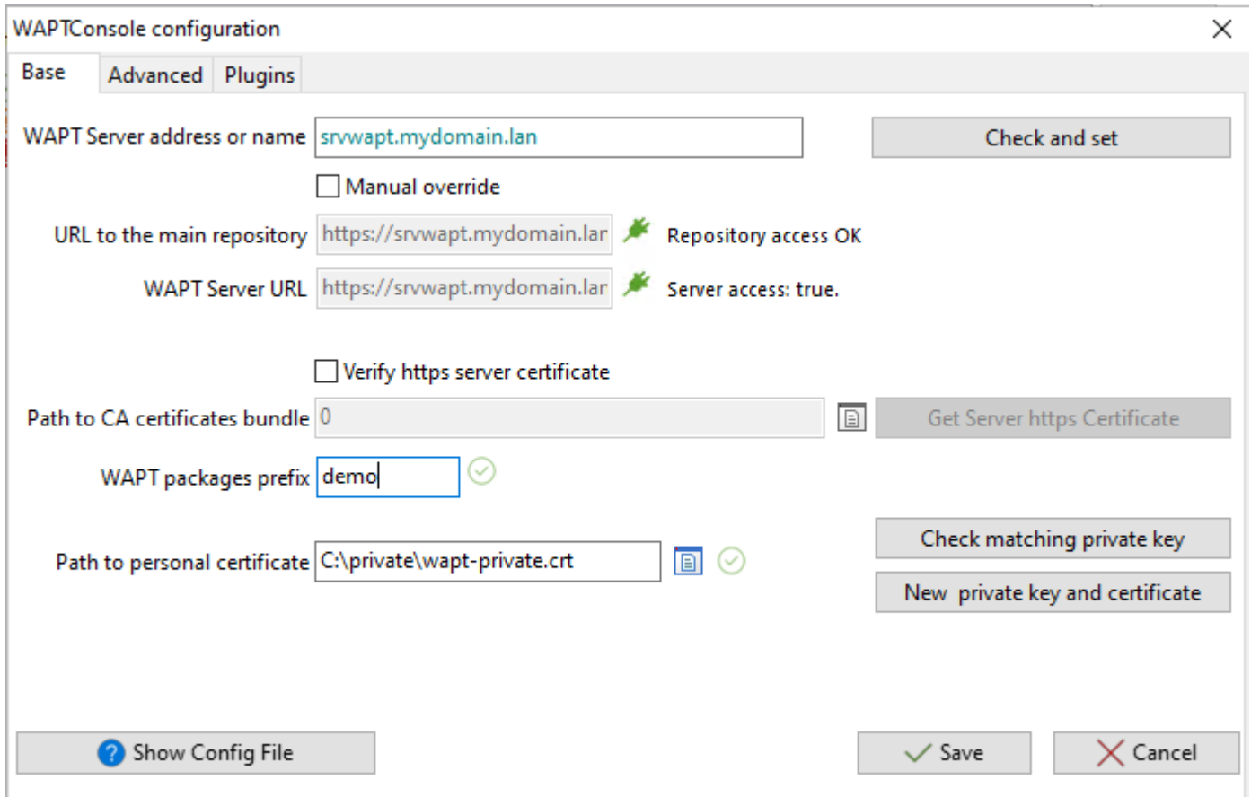
FIG. 8 – Fenêtre pour la configuration basique de la console WAPT
