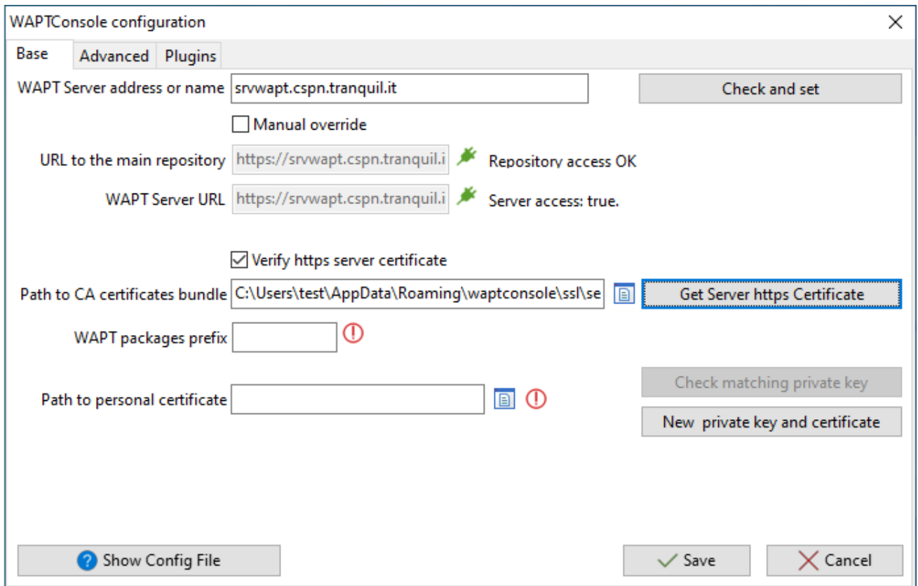
FIG. 8 – La configuration de la console WAPT SSL est OK
